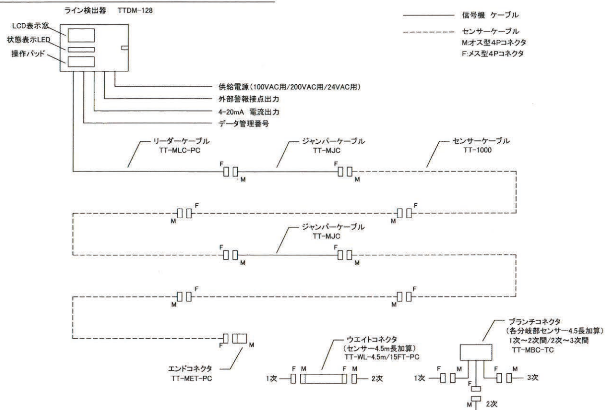
トレーステック・ライン検出システム・システム構成図
